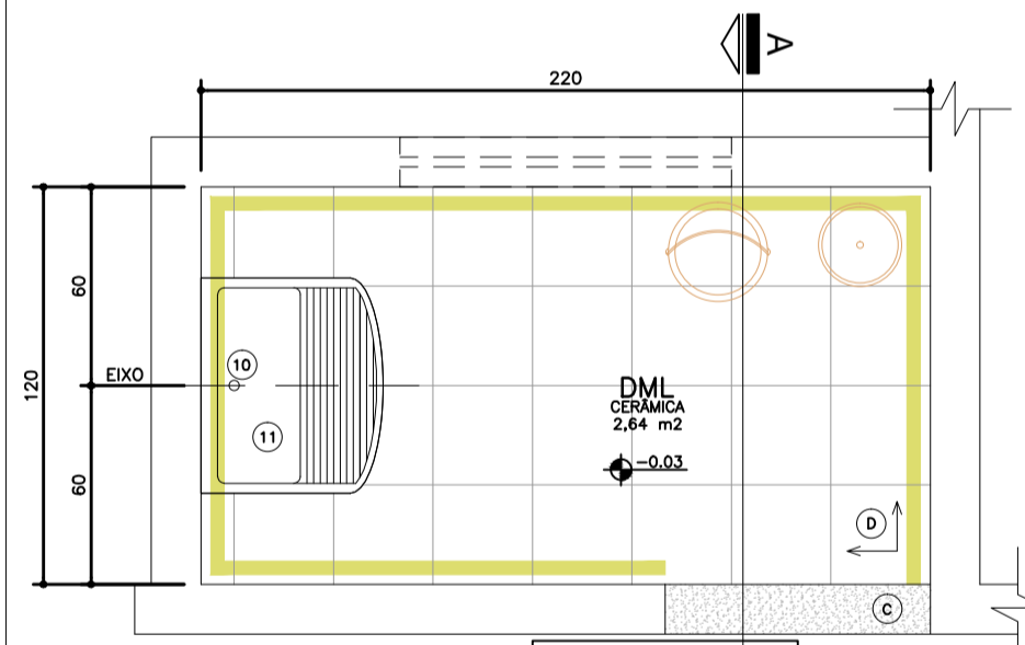
01 Planta Baixa Amb. 01 - DML Esc.: 1:25
