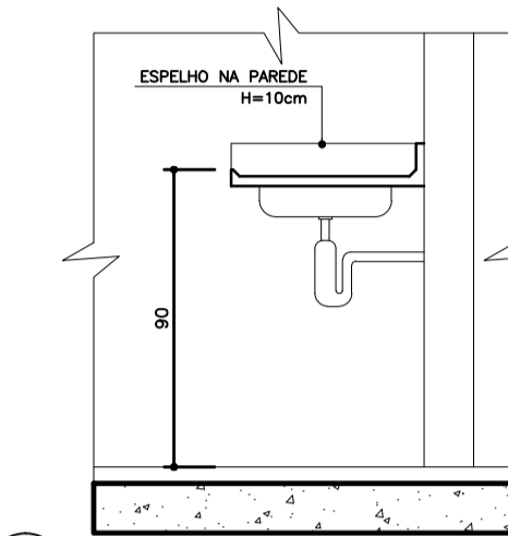
09 Detalhe 1 Esc.: 1:25
