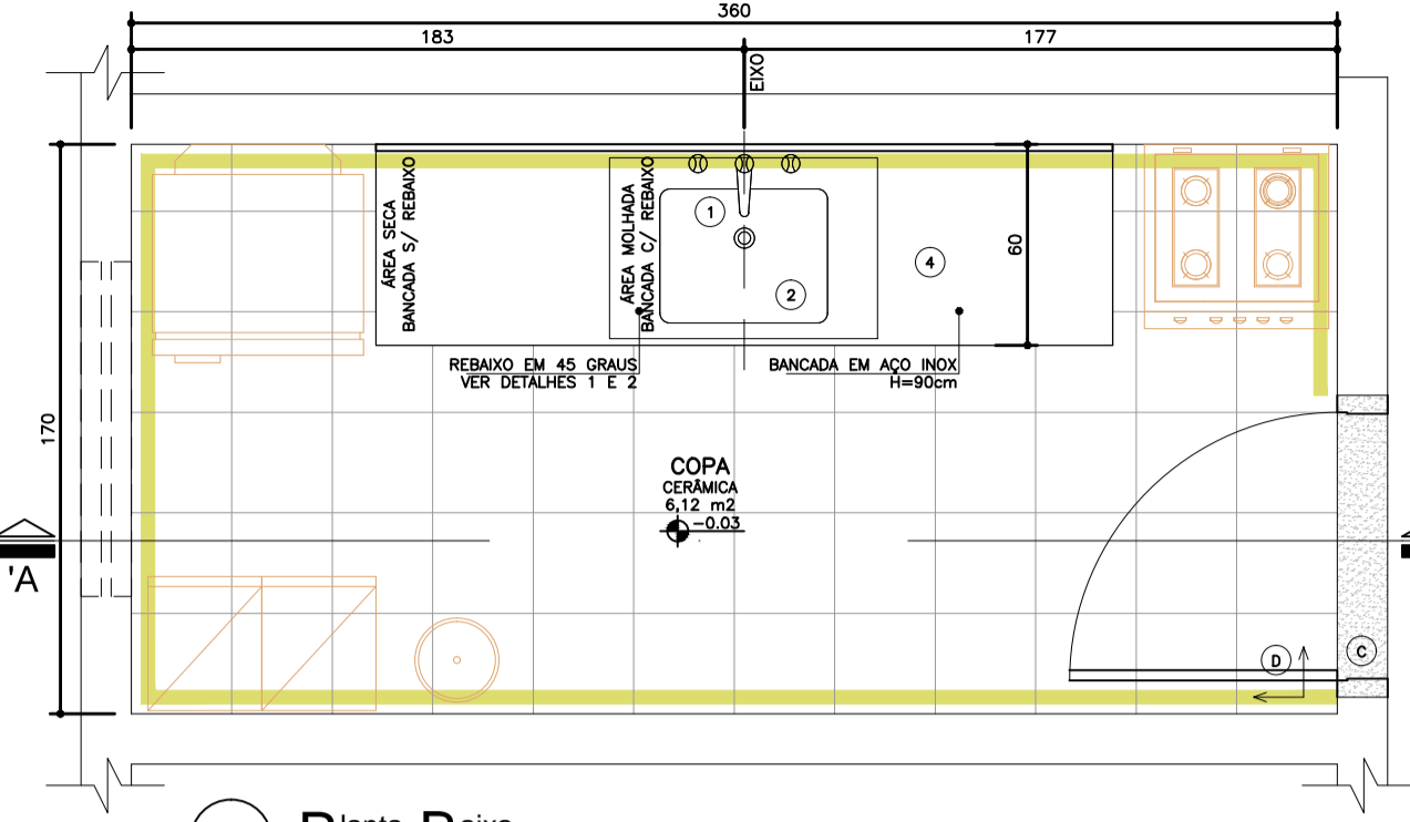
07 Planta Baixa Amb. 04 - COZA Esc.: 1:25
