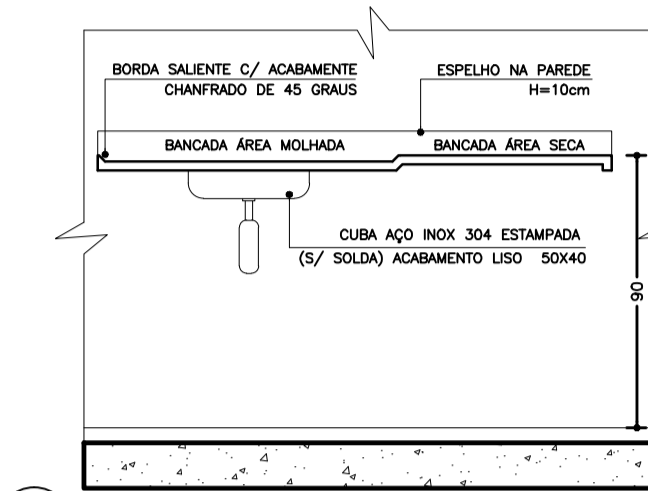
10 Detalhe 2 Esc.: 1:25
