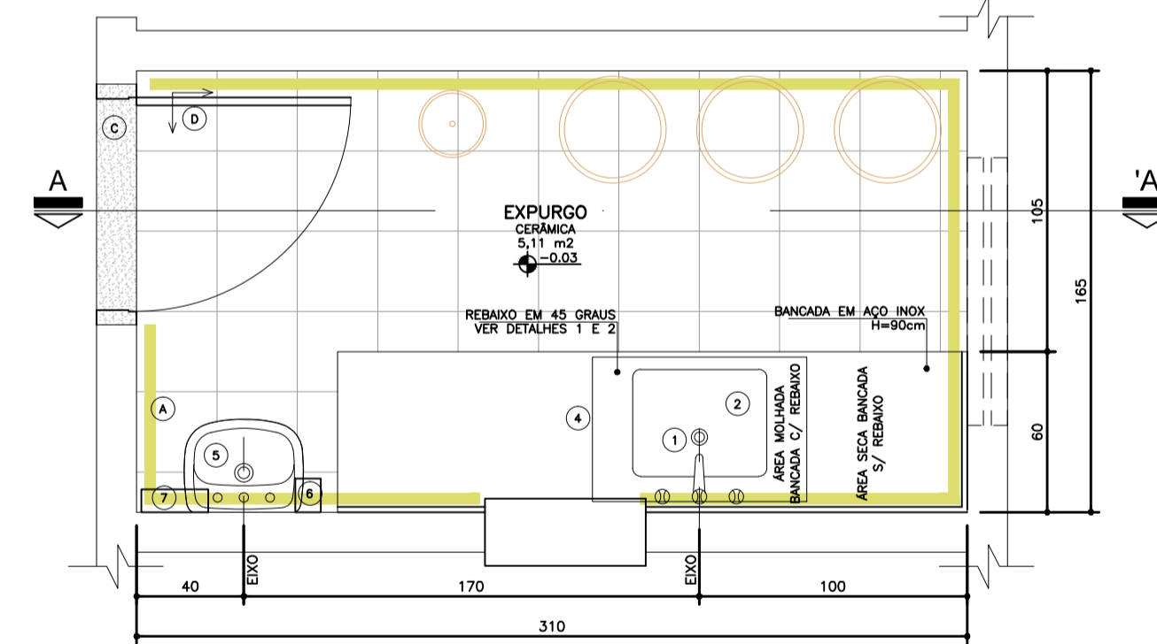
03 Planta Baixa Amb. 02 - EXPURGO Esc.: 1:25
