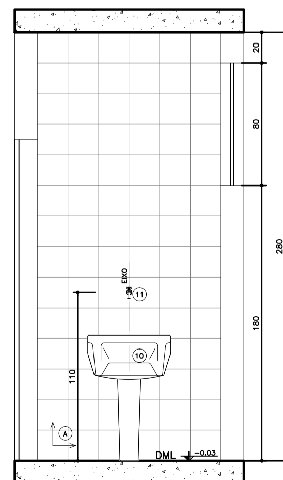
02 Seção AA' Amb. 01 - DML Esc.: 1:25
