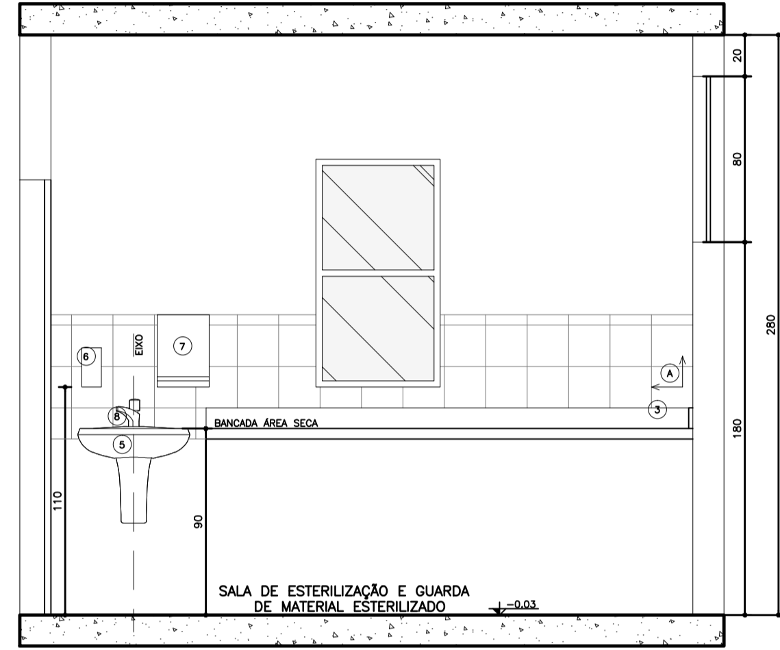
06 Seção AA' Amb. 03 - Esterilização Esc.: 1:25
