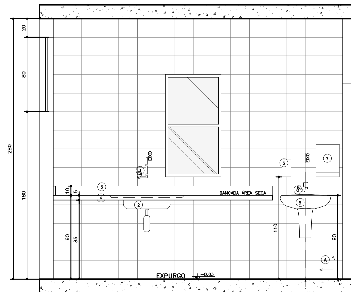
03 Planta Baixa Amb. 02 - EXPURGO Esc.: 1:25
