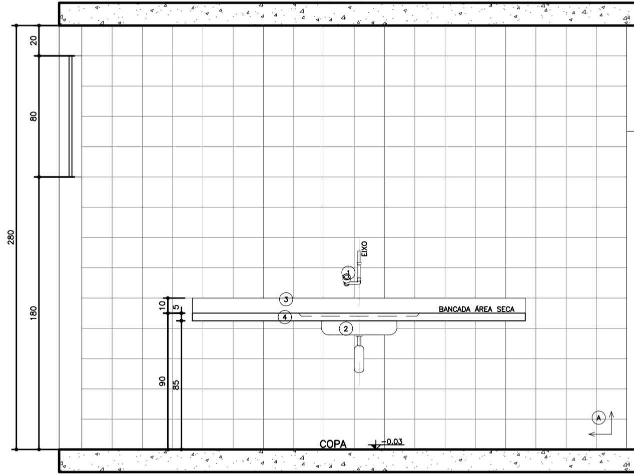
08 Seção AA' Amb. 04 - Coza Esc.: 1:25
